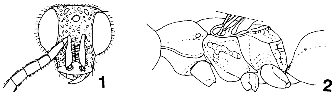
図1, 2. トゲナナフシバチ Calosega kamiteta Terayama, 1999, オス 1, 頭部, 正面観 ; 2, 胸部, 側面.
